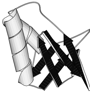
OB Fold
