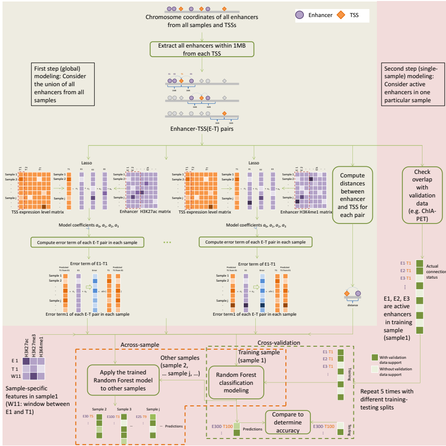
Figure S 3-11 (TL, #) Schematic of JEME
