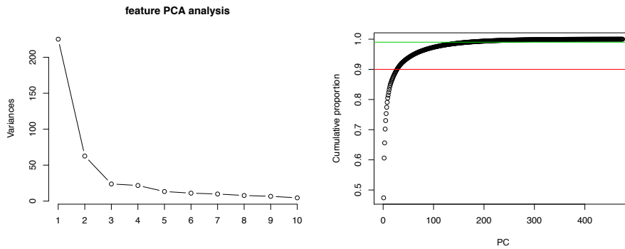
Figure S 2-7 (TL, #) Summary of feature PCA analysis
