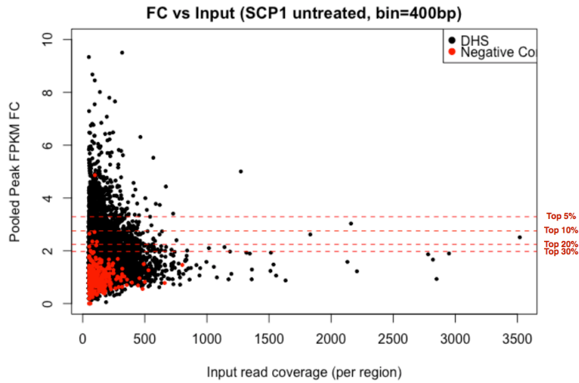
Figure S 3-10 (TL, #) Capture STARR-seq experiment properties
