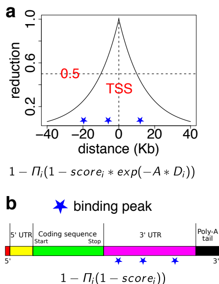
Figure S 4-3. (TL, #) Regulatory network construction
