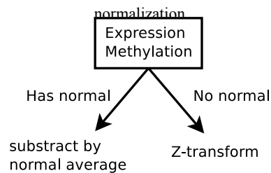
Figure S 4-2 (TL, #) Schematic of RNA-seq
