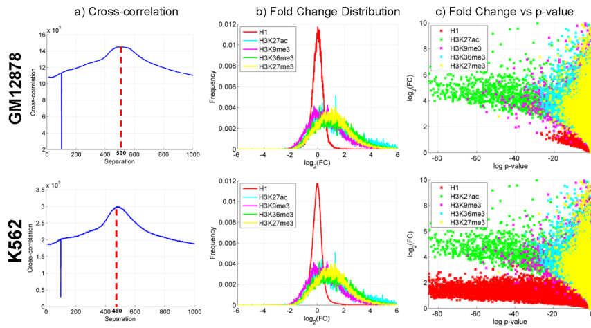
Figure S 3-10 (TL, #) Capture STARR-seq experiment properties
