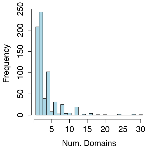
b) Domains
