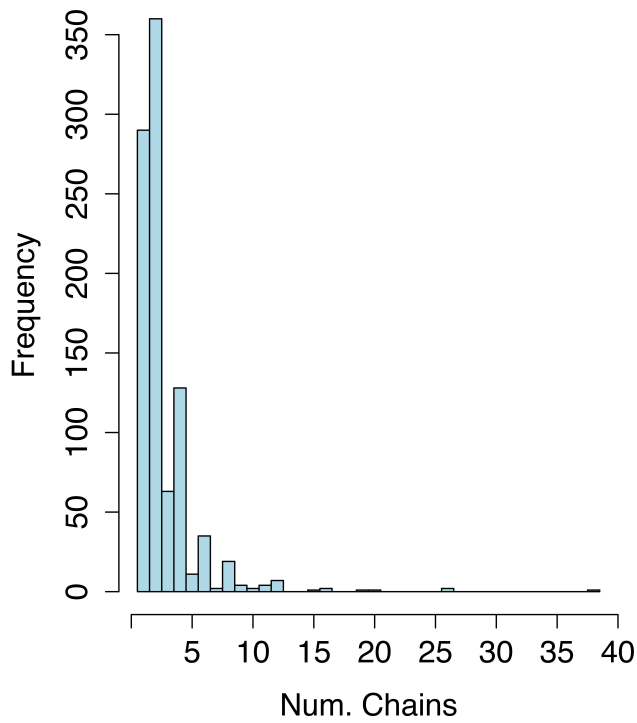
a) Chains
