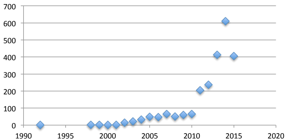
Eucaryotes - # species
