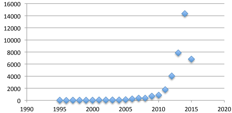
Prokaryotes - #species
